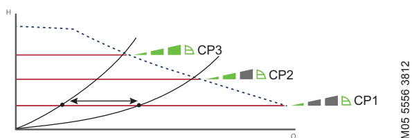
Fig. 8 Tre curve/impostazioni a pressione costante
