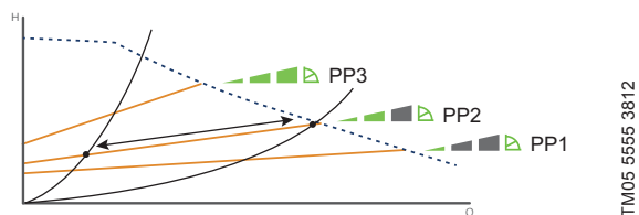
Fig. 7 Tre curve/impostazioni a pressione proporzionale
