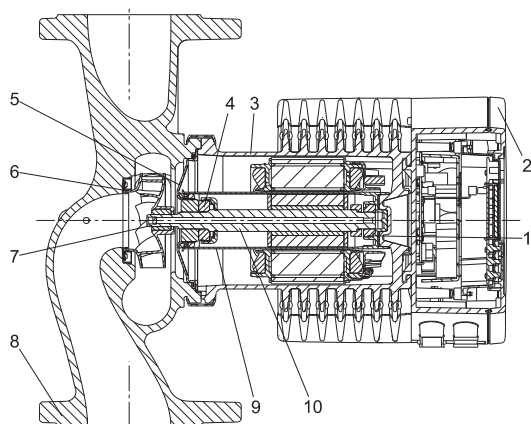
Fig. 13 Versione flangiata con canotto separatore in PPS-composito.
