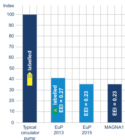
Fig. 23 Indice di consumo energetico
