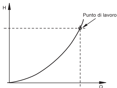
Fig. 5 Caratteristica dell'impianto
