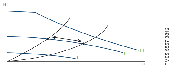
Fig. 9 Tre impostazioni di curva costante/velocità costante
