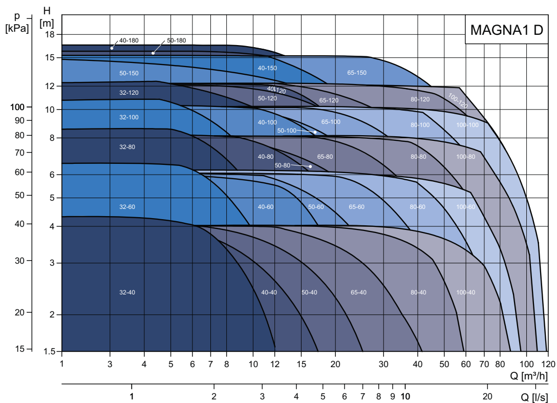
Fig. 4 Gamma delle prestazioni, funzionamento gemellare MAGNA1 D
